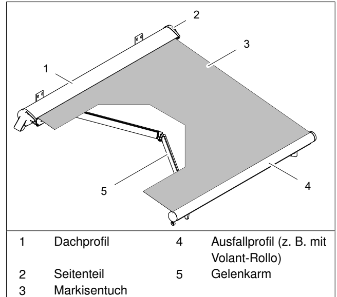
Abb. 1: Gelenkarm-Markise H60/G60 (abgebildet H60)
